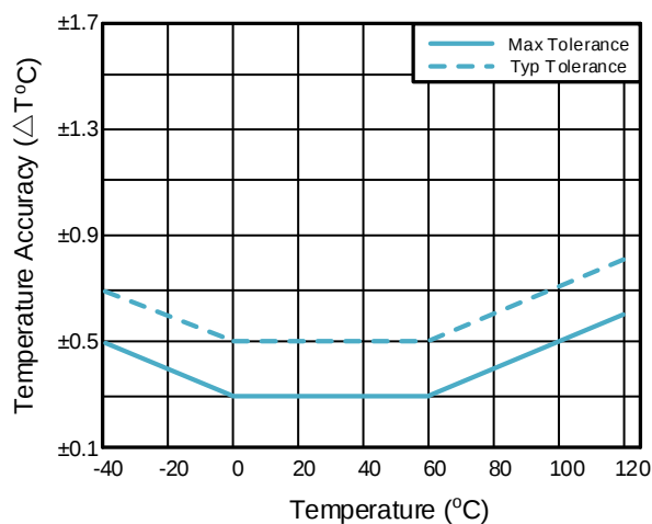
图 2. GD30TSHTC3 温度误差
