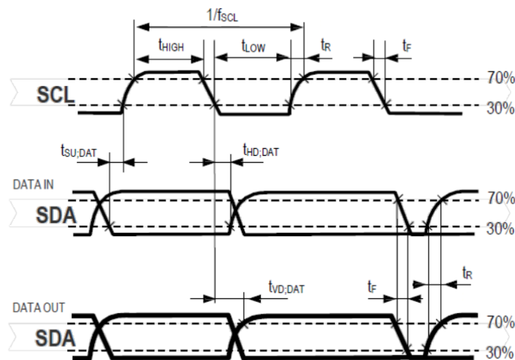
图 6. 输入输出 pad 的时序图
