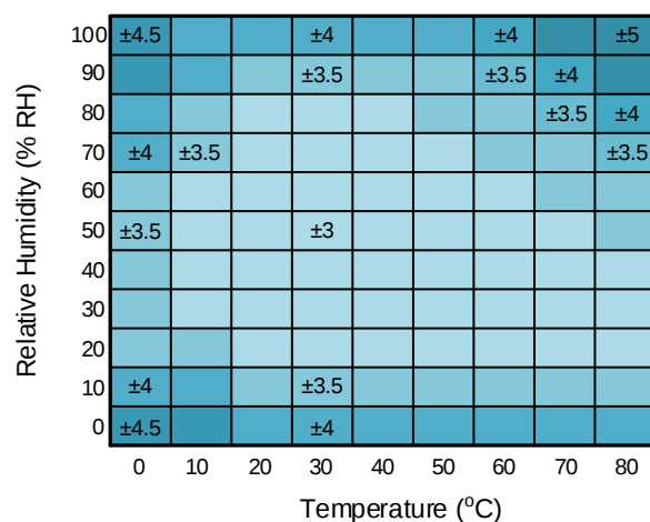
图 3. GD30TSHTC3 不同温度条件下的相对湿度典型误差
