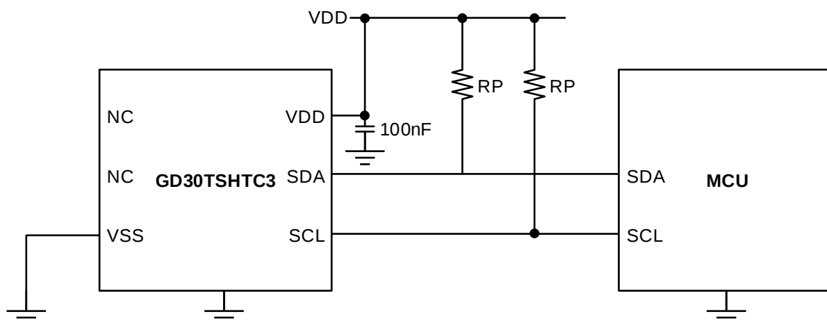
图 7. GD30TSHTC3 典型参考电路
