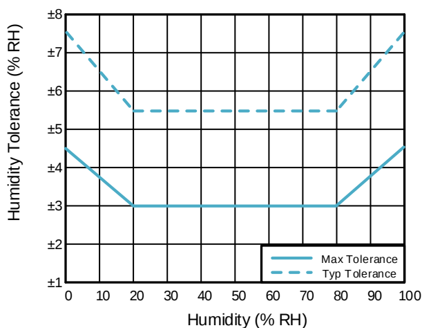
图 1. GD30TSHTC3 湿度误差@25°C
